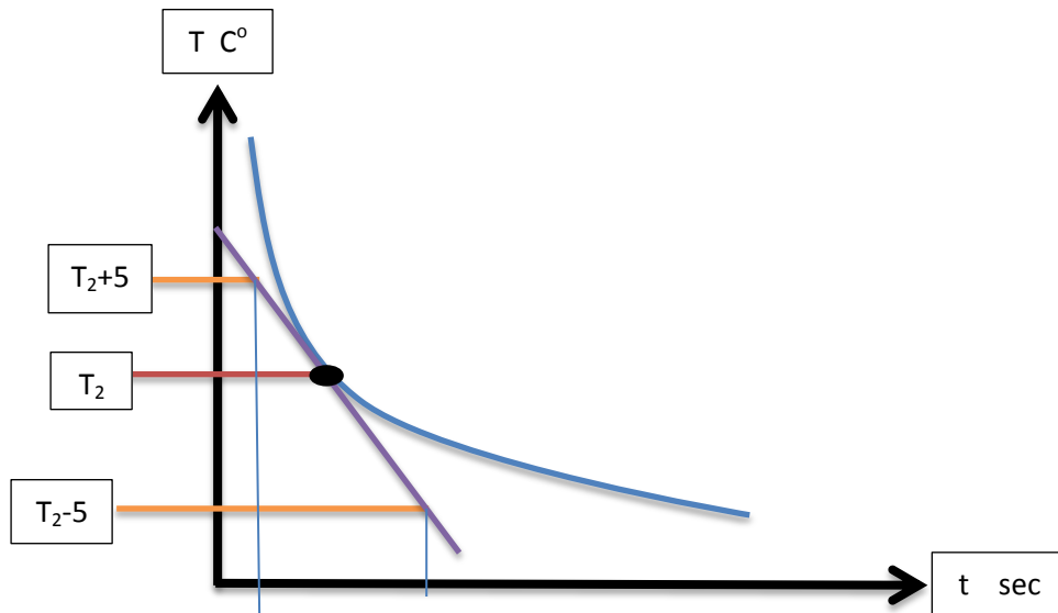
شكل (2) منحني التبريد
