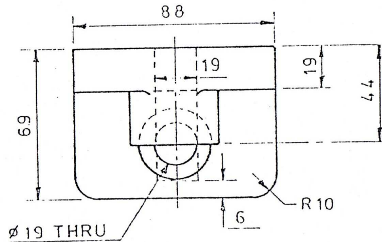
تمرين 3.73 مستند منزلق - المادة : حديد صلب
