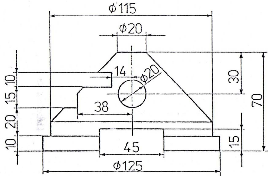
تمرين 3.74 مخروط - المادة : فولاذ
