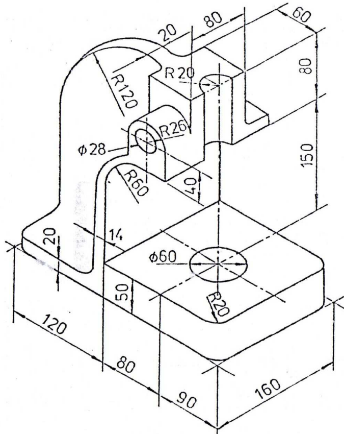
تمرين 3.50 مكبس - المادة : حديد صلب
