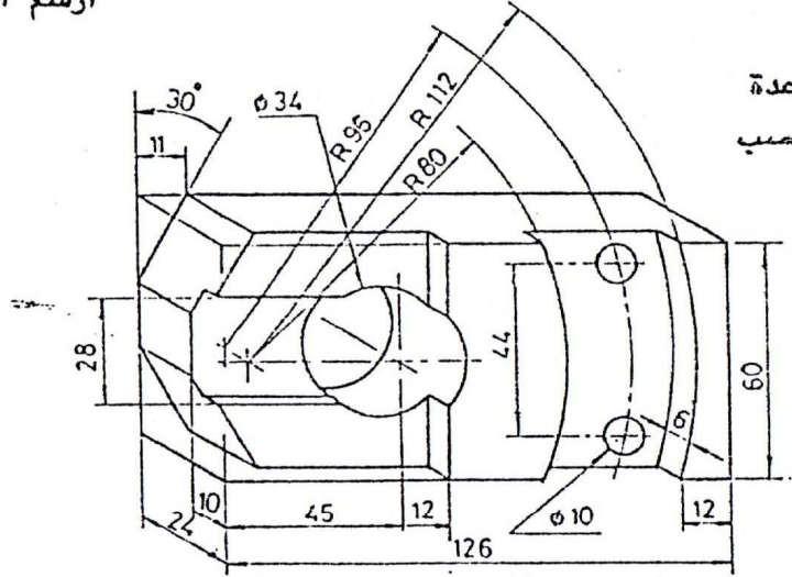
تمرين 3.49 مؤشر - المادة : فولاد
